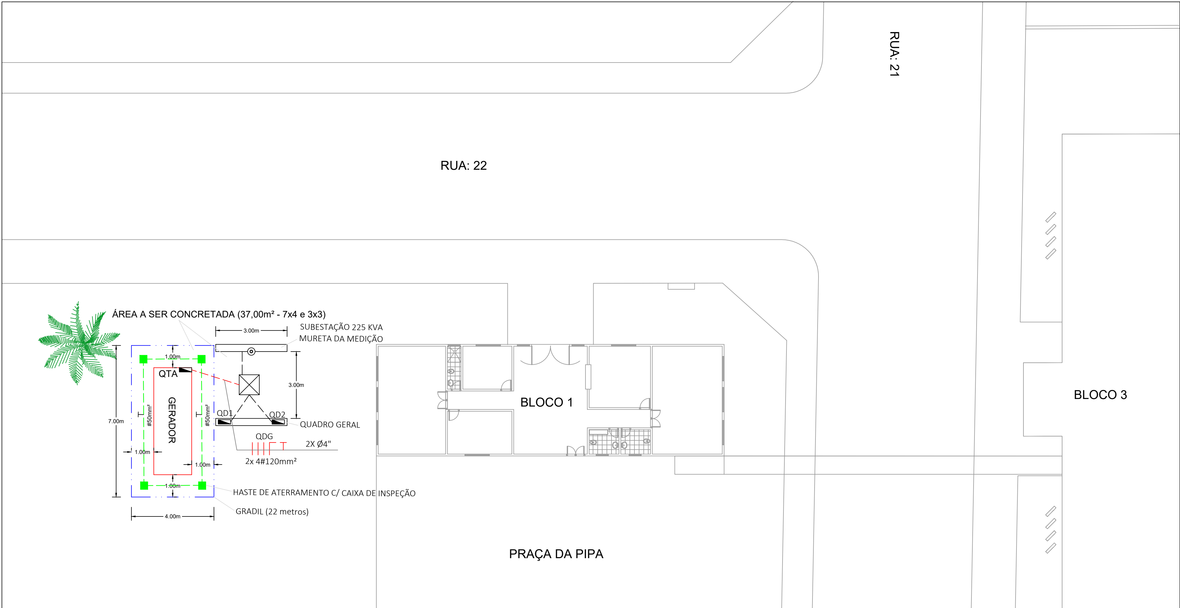
PLANTA BAIXA ESCALA: 1/100
