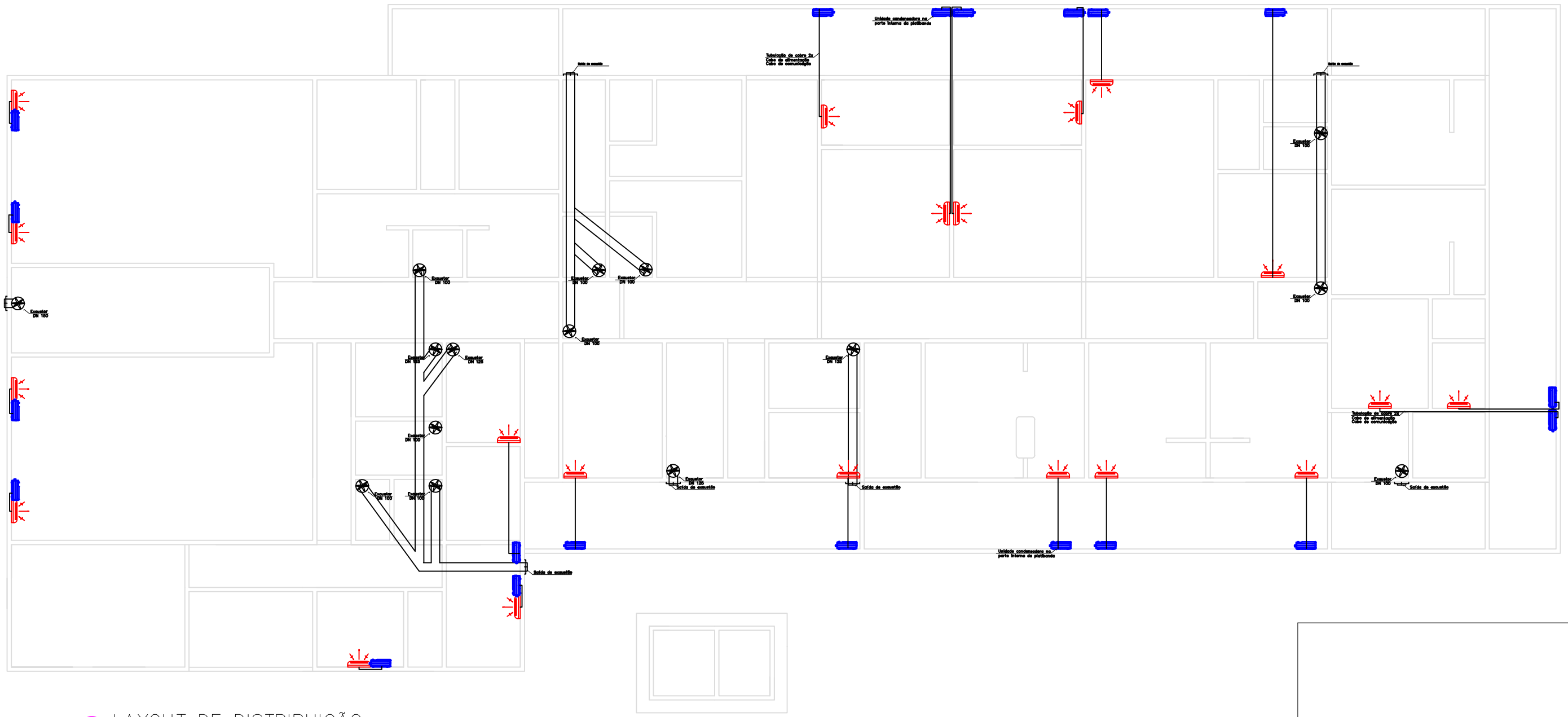
1 LAYOUT DE DISTRIBUIÇÃO ESCALA -1 : 150
